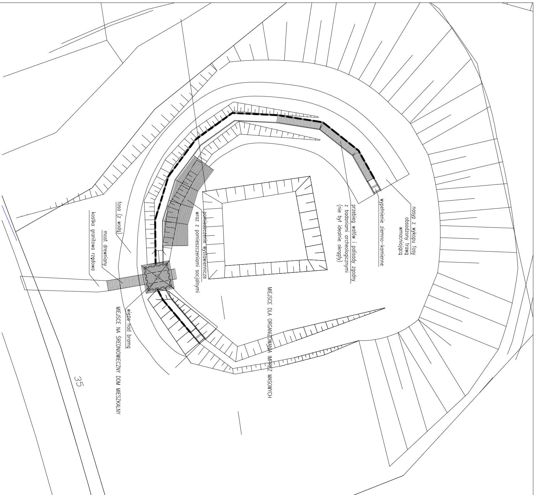
RZUT GRODU 1:500
